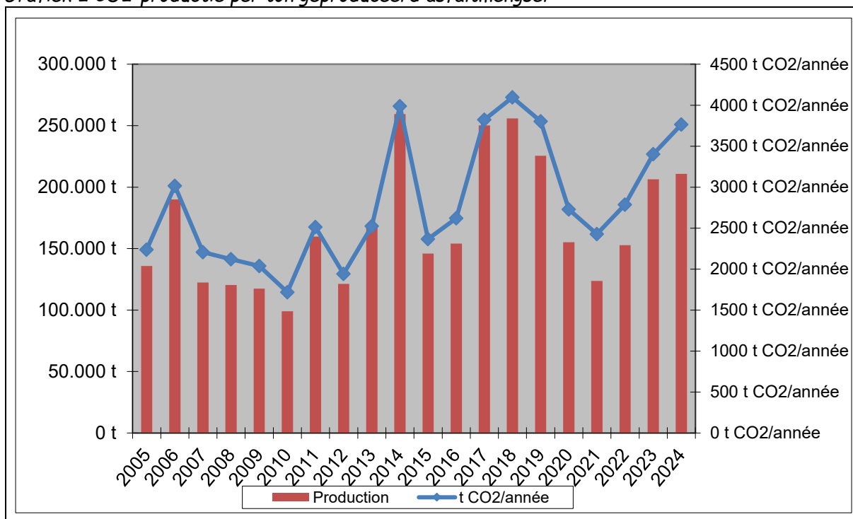
Grafiek 2 CO2-productie per ton geproduceerd asfaltmengsel
