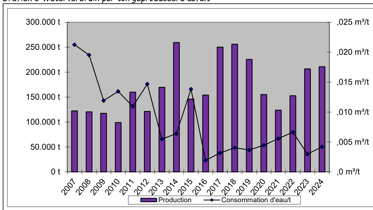
Grafiek 3 Waternverbruik per ton geproduceerd asfalt
