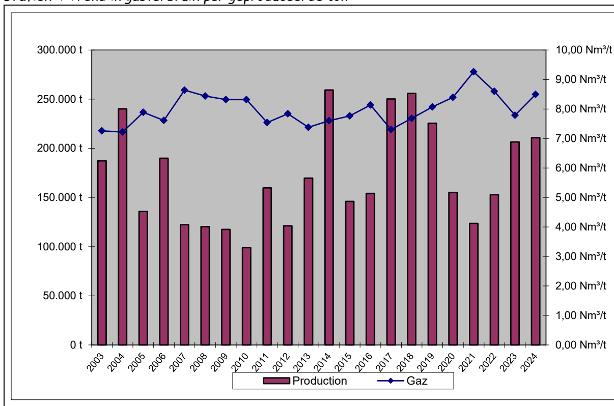
Grafiek 4 Trend in gasverbruik per geproduceerde ton
