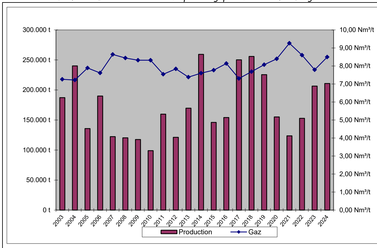
Grafiek 5 Elektriciteitsverbruik per ton geproduceerd asfaltmengsel
